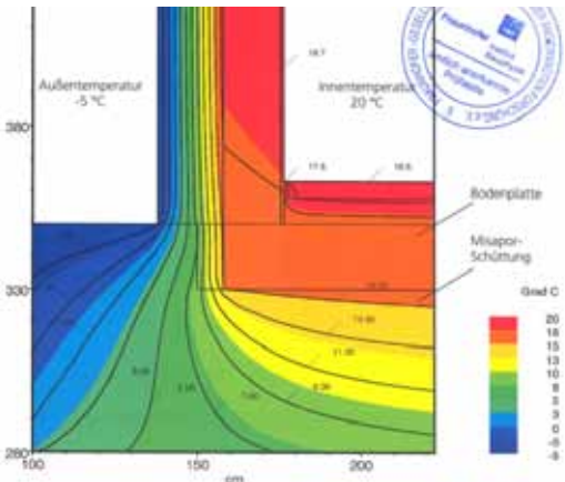
Extrait du rapport de test P7-101/2009, détail avec calcul du passage thermique avec le remblai( avec le Lambda 0.085 W/(m*K)), est de l'institut Fraunhofer pour la physique du bâtiment
