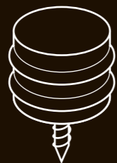
butoir de porte 32 mm diamètre 34 mm hauteur
